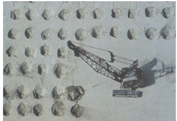
10.2. ábra. Dinamikus konszolidáció.
