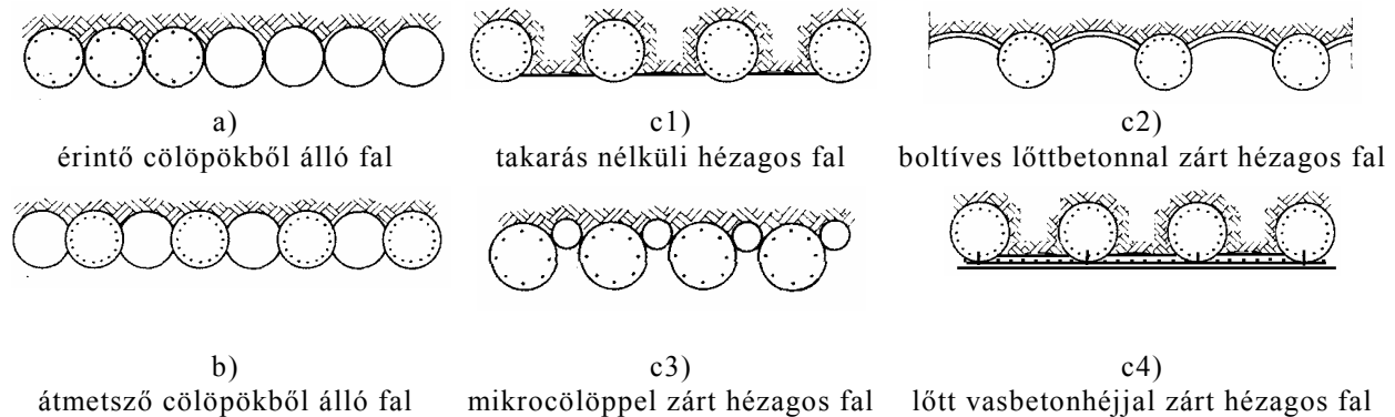
8.12. ábra. Cölöfaltípusok.
