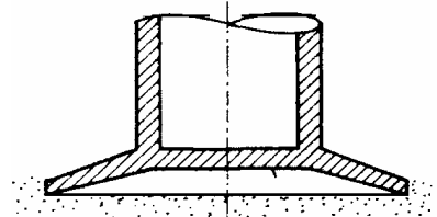
6.7. ábra. Dobozalap.
