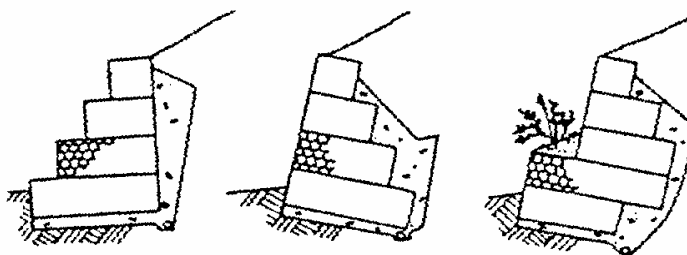
8.21. ábra. Gabionfalak.
