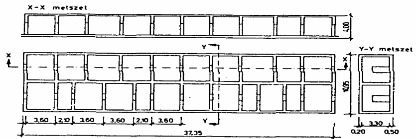
6.7. ábra. Dobozalap.
