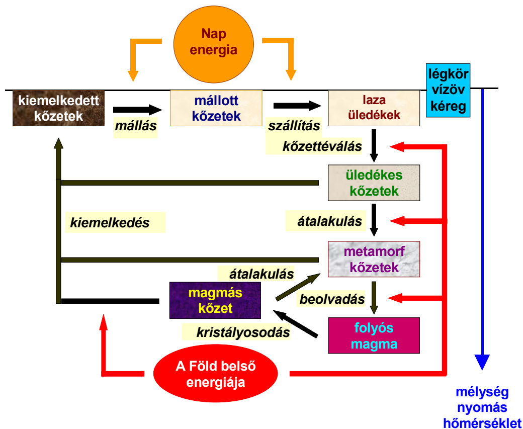
1.3. ábra A kőzetciklus.
